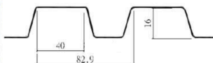
鋼板成型斷面圖
